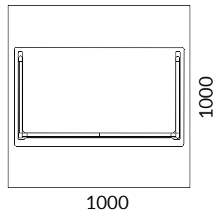
Draufsicht (mit Counter Top)
